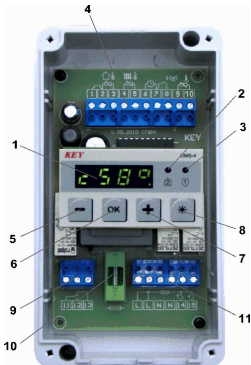
Rysunek 1. Widok płyty czołowej modułu UMS-4PRh.
