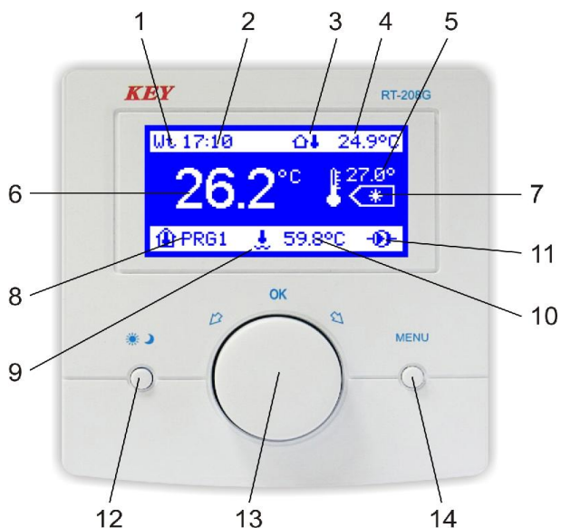
Рис.1. Лицевая панель регулятора RT-208G.
