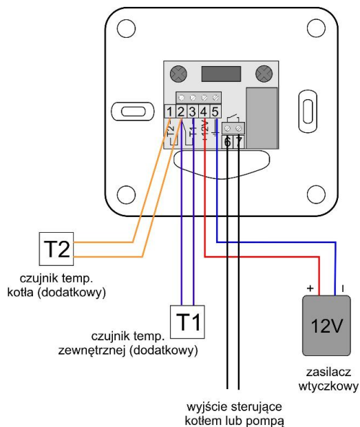
Схема подключения регулятора RT-208G с двухжильным кабелем для котла или регулятора насоса СН (мощность насоса до 200 Вт / 230 В).
