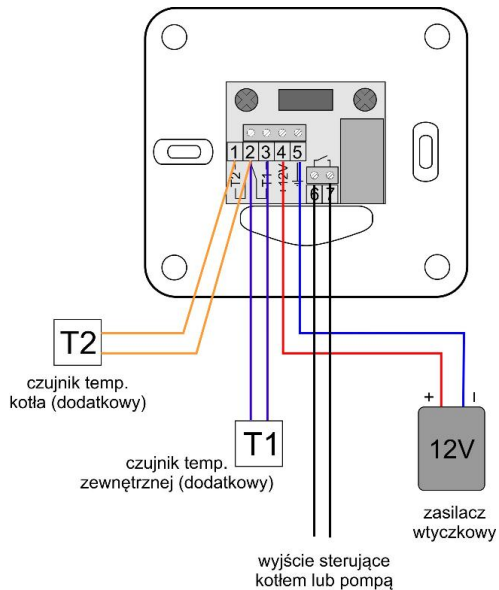
Schemat podłączenia regulatora RT-208G przewodem dwużyłowym do regulatora kotła lub pompy CO (moc pompy do 200W / 230V)
