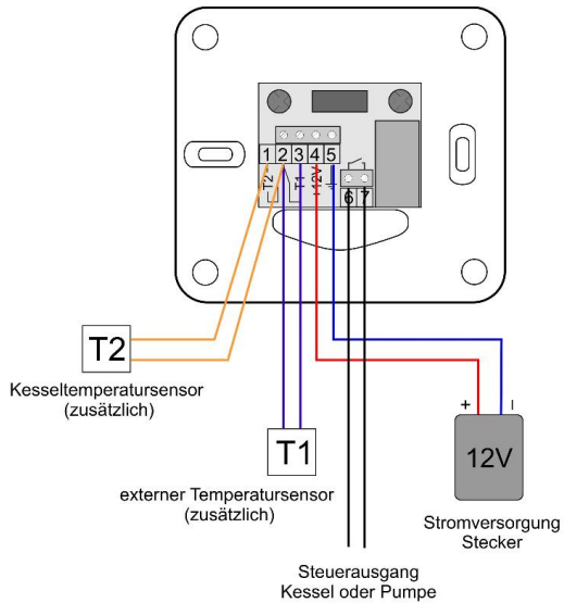
Anschlussplan des Reglers RT-208G mit einem zweiadrigen Kabel für einen Kessel oder CH-Pumpenregler (Pumpenleistung bis 200W / 230V)
