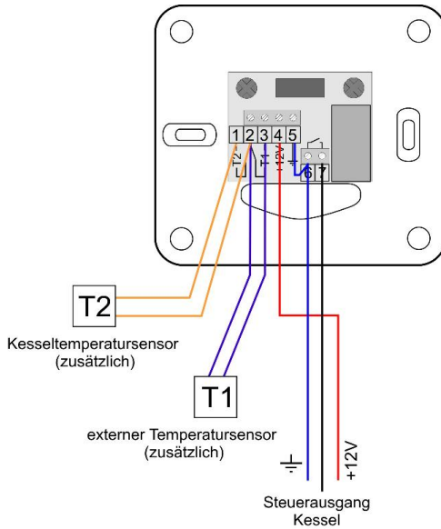
Anschlussplan des Reglers RT-208G mit einem zweiadrigen Kabel für einen Kessel oder CH-Pumpenregler (Pumpenleistung bis 200W / 230V)
