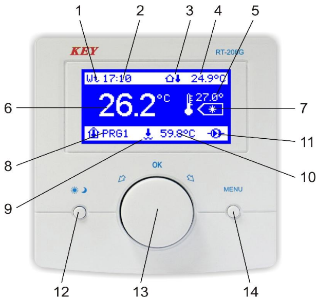
Abbildung 1. Frontplatte des Reglers RT-208G.
