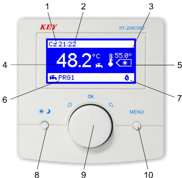
Rysunek 1. Płyta czołowa regulatora RT-208CWU.
