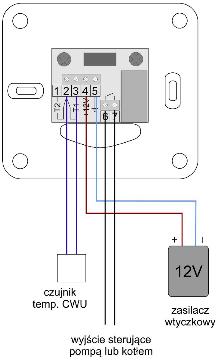
Rysunek 2. Schemat podłączenia regulatora RT-208CWU.
