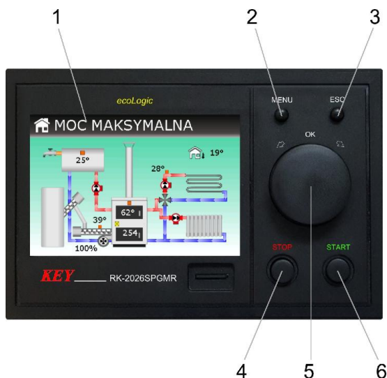
Rysunek 1. Płyta czołowa regulatora RK-2026SPGMR.
