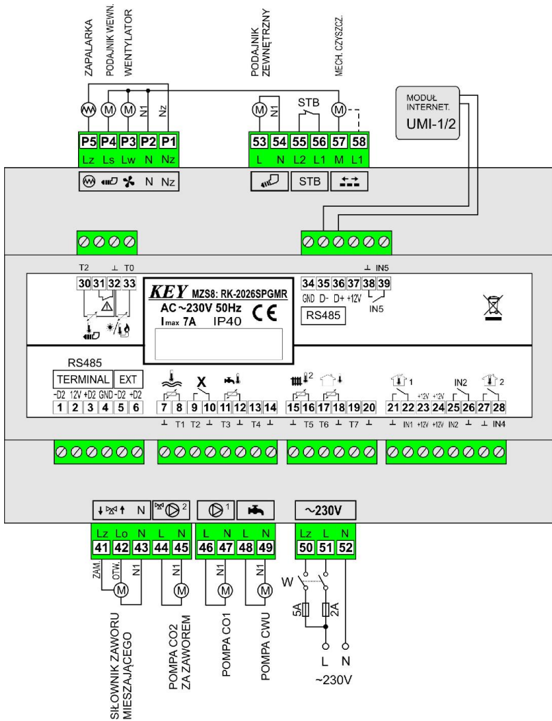
Rysunek 3. Schemat podłączenia RK-2026SPGMR+MZS8/MZM8.
