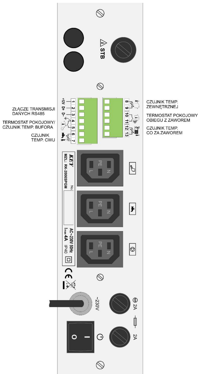
Schemat podłączenia regulatora RK–2006SPGMA z modułem zasilacza M.ZL.
