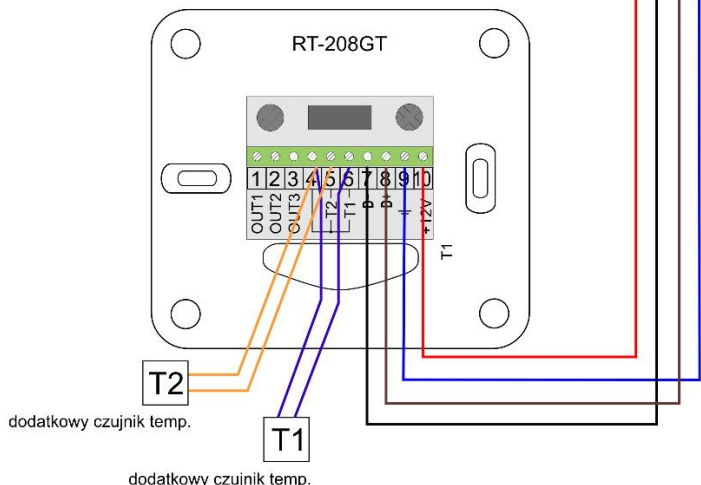
Schemat podłączenia regulatora RT-208GT do regulatora RK-2006SPGMA z modułem zasilacza MZK, MZM2.
