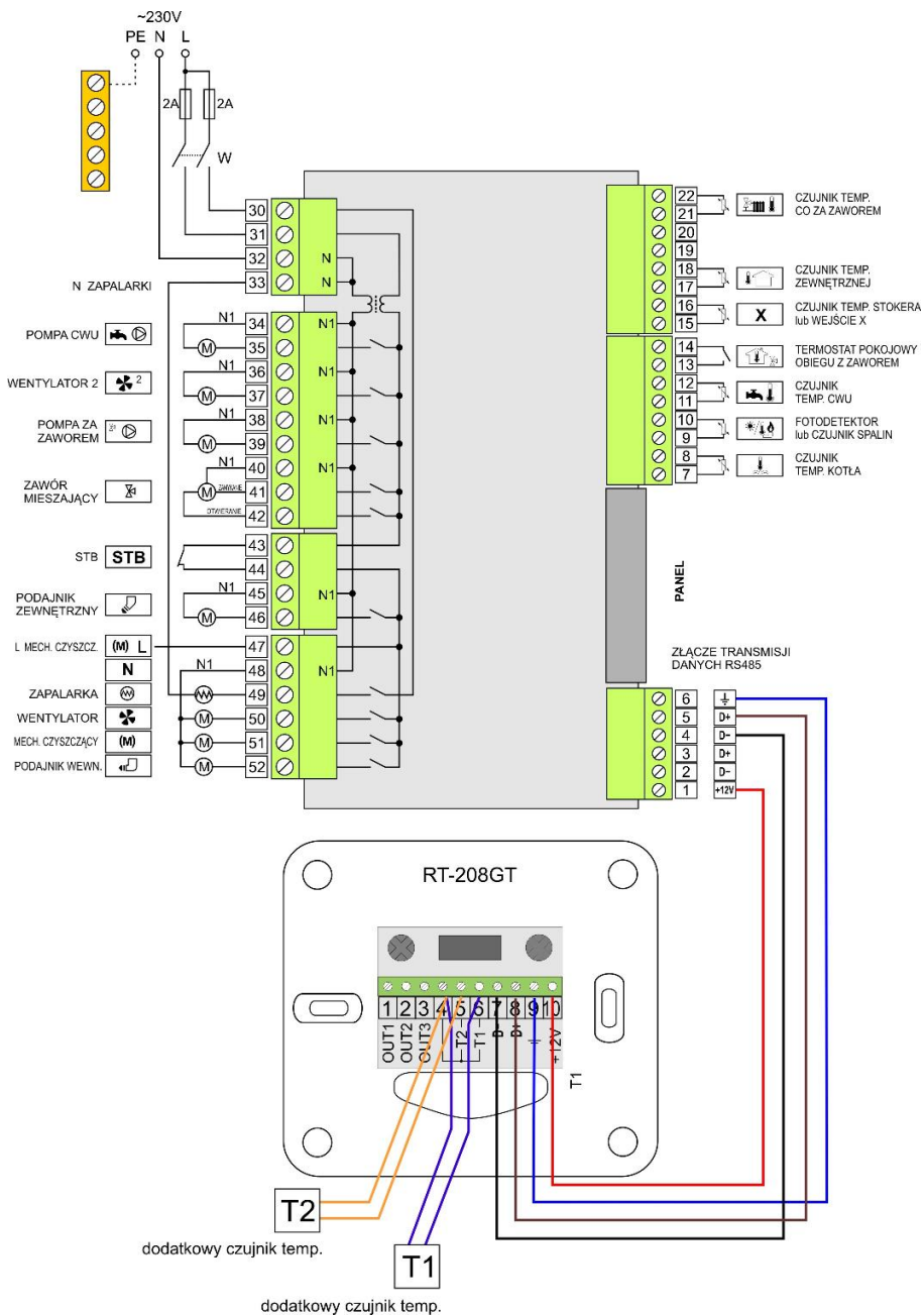
Rysunek 3. Schemat podłączenia regulatora RT-208GT z modułem zasilacza MZK4, MZM wersja V.06.2015.
