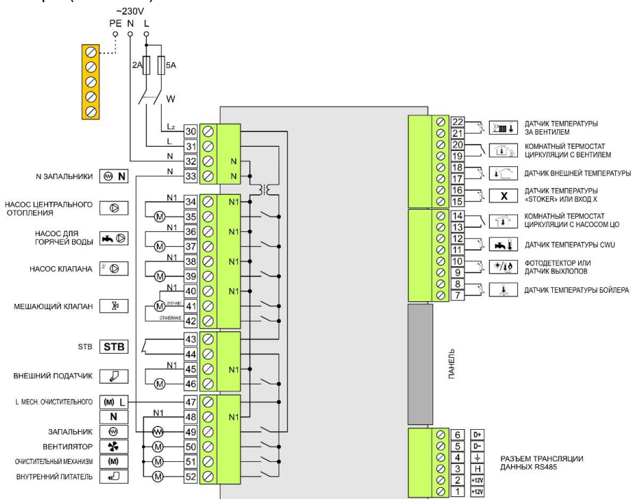
Схема подключения регулятора RK-2006SPGM+MZK, MZM2
