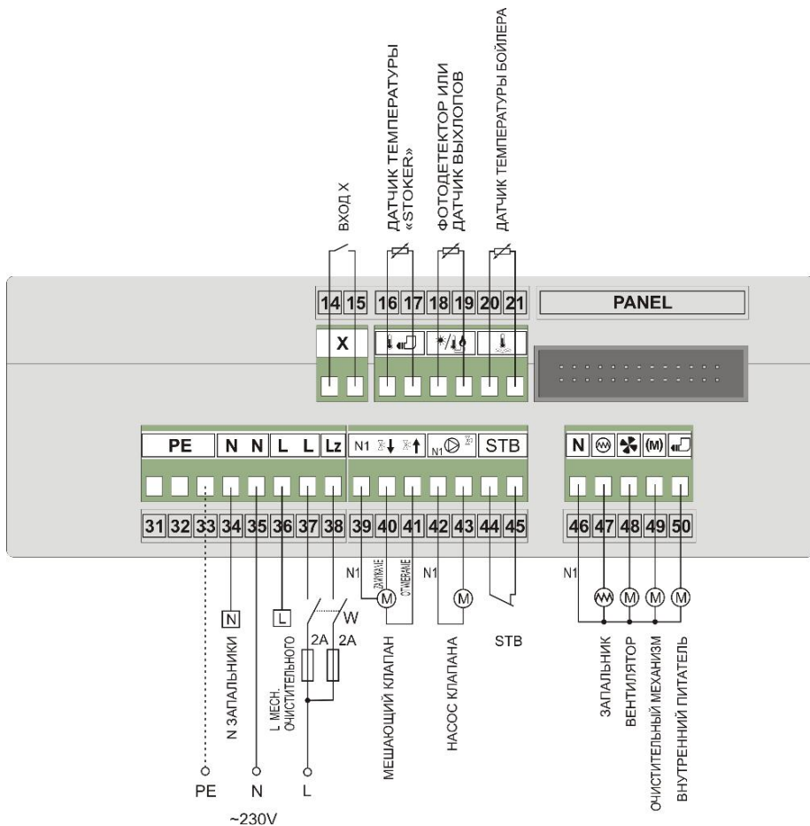
Схема подключения регулятора RK-2006SPGM+MZL.
