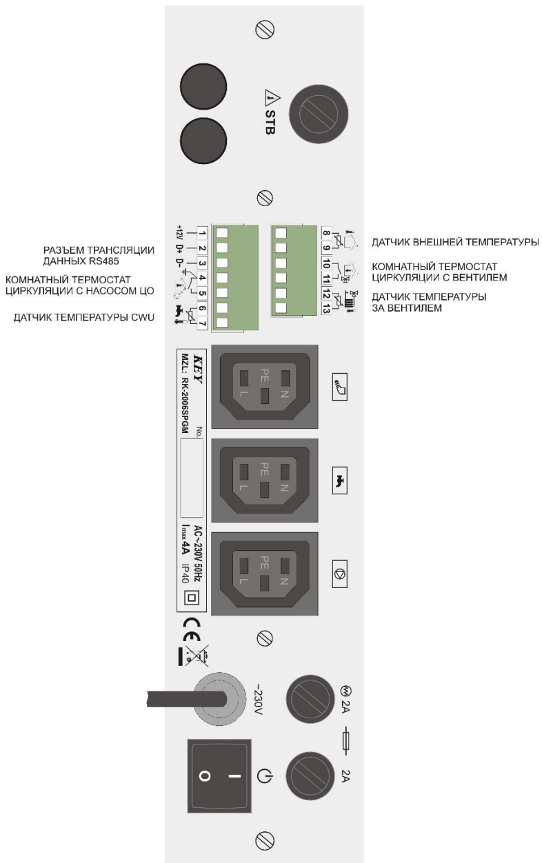
Схема подсоединения регулятора RK-2006SPGM+MZL.
