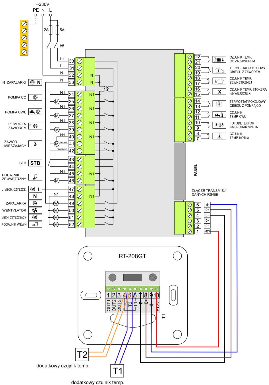
Schemat podłączenia regulatora RT-208GT do regulatora RK-2006SPGM z modułem zasilacza MZK, MZM2 wersja V.06.2015
