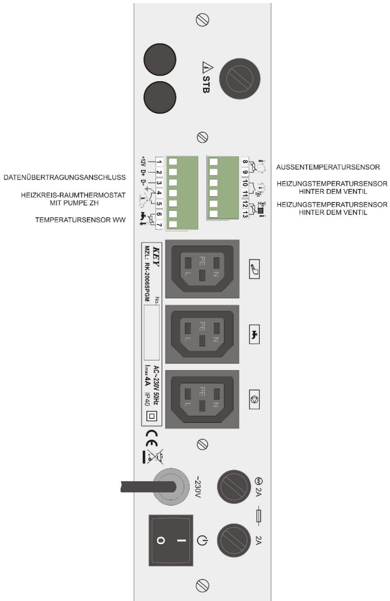
Anschluss Schaltplan des Reglers RK-2006SPGM mit Netzgerät MZL Version V.06.2015
