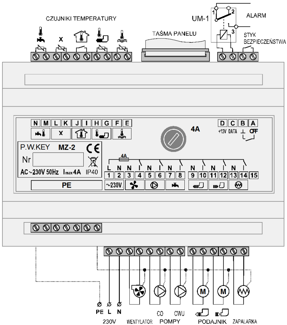
Rysunek 3. Schemat podłączenia modułu zasilacza regulatora RK-2006LSH.
