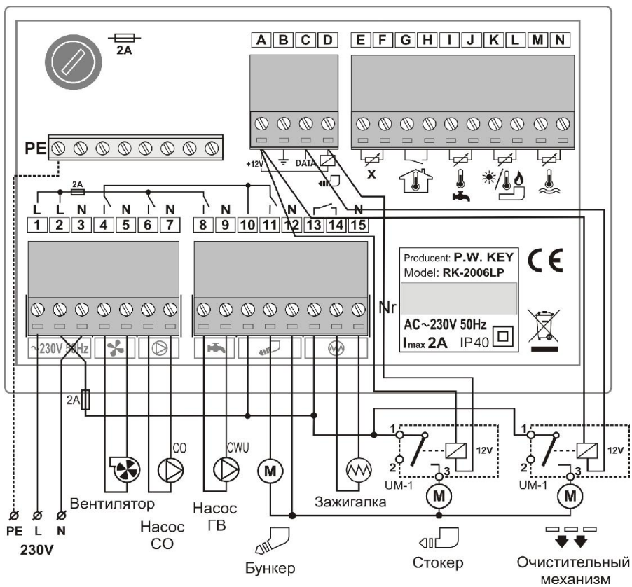
Рис. 2. Диаграмма подключения контроллера RK-2006LPP.
