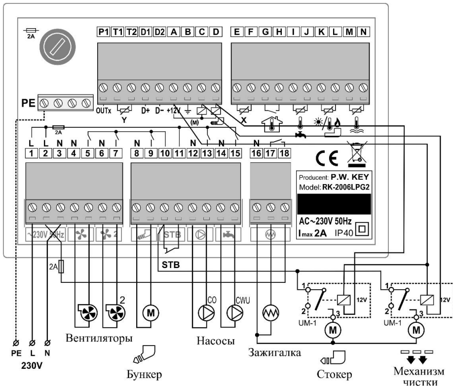
Рисунок 2. Схема подсоединения регулятора RK-2006LPG2.
