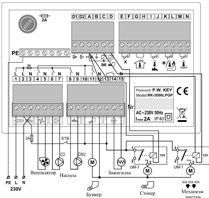
Рисунок 2. Схема подсоединения регулятора RK-2006LPGP.
