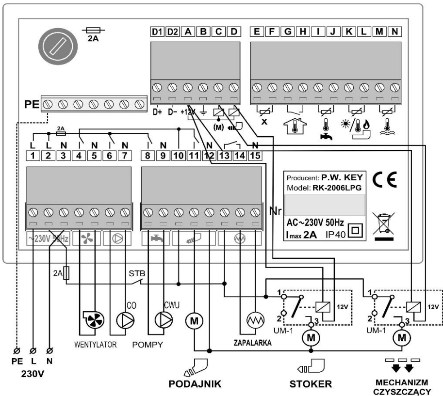
Rysunek 2. Schemat podłączenia regulatora RK-2006LPGD.
