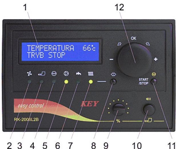
Рис. 1. Передняя панель контроллера RK-2006L2B
