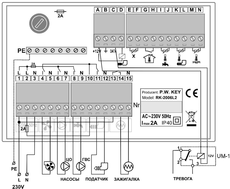
Рисунок 4. Схема подключения регулятора RK–2006L2 (с системой сигнализатора тревог).
