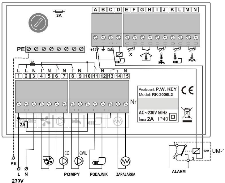
Rysunek 4. Schemat podłączenia regulatora RK-2006L2.
