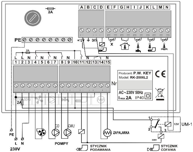
Rysunek 3. Schemat podłączenia regulatora RK-2006L2 z układem cofania paliwa.
