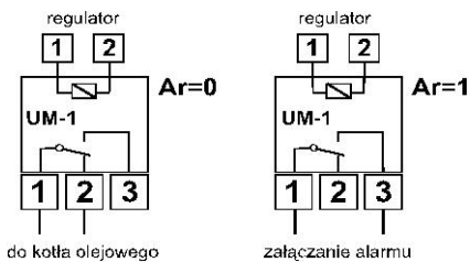
Rysunek 4. Schematy podłączenia modułu UM-1.
