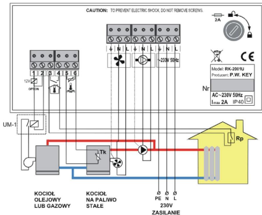
Rysunek 3. Schemat podłączenia regulatora RK-2001U.
